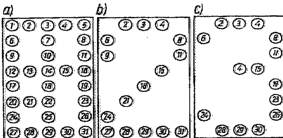
Rys. W.30. Wskaźniki cyfrowe elektryczne (światłne): a) pełny układ punktów światlnych, b) i c) przykłady utworzenia cyfr 2 i 3 [7]
